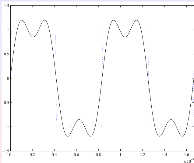
Slika: Pravokutni signal ( f = 1200 Hz) propušten kroz idealni AA filtar.
