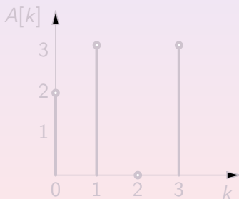
Slika: Amplitudni spektar
