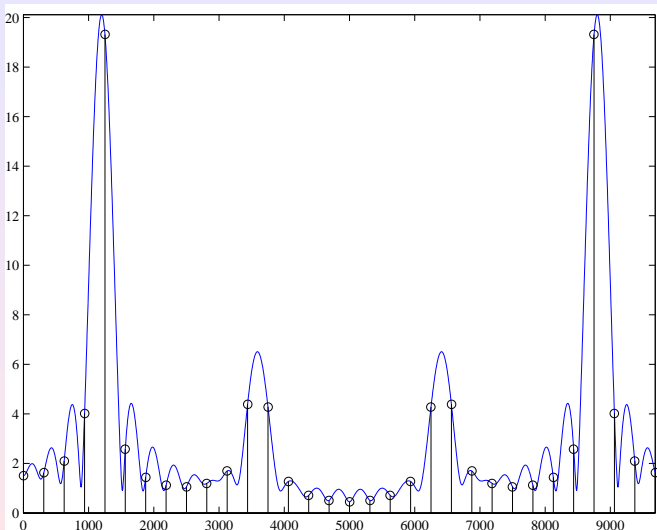
Slika: Spektar signala uz N = 32 , frekvencijska os u Hz.
