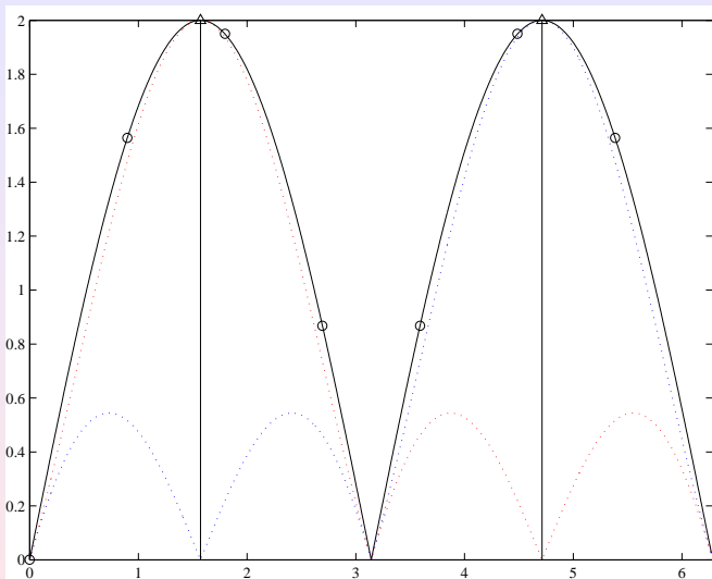
Slika: Amplitudni spektar (DFT i DTFT) za P = L = 4 , N = 7
