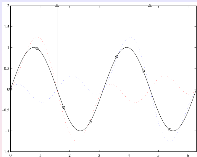
Slika: Imaginarni dio spektra za P = L = 4 , N = 7
