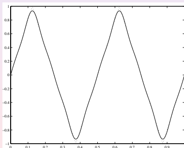
Slika: Trokutasti signal
