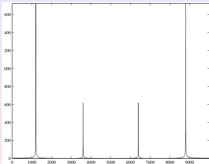
Slika: Spektar signala uz N = 4096 , frekvencijska os u Hz.
