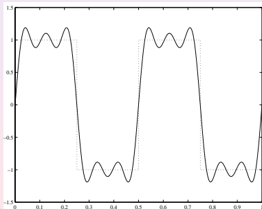
Slika: Pravokutni signal
