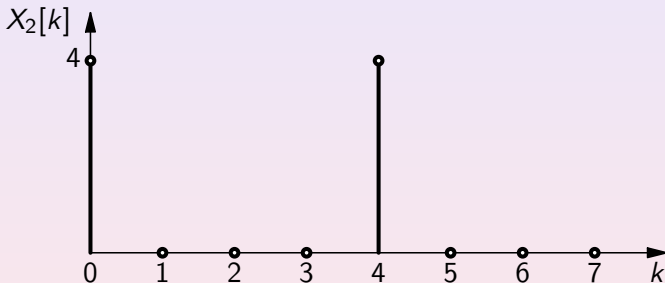
Slika: Amplitudni spektar X_2[k]
