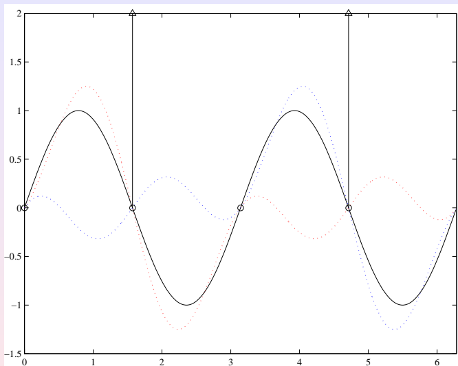
Slika: Imaginarni dio spektra za P = L = N = 4
