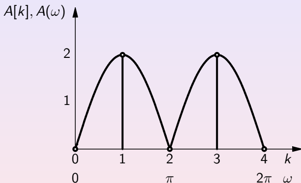
Slika: Amplitudni spektar (DFT i DTFT)
