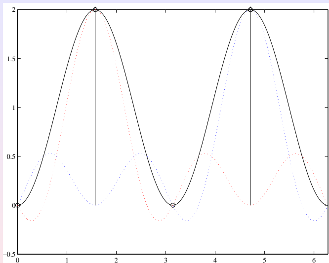
Slika: Realni dio spektra za P = L = N = 4
