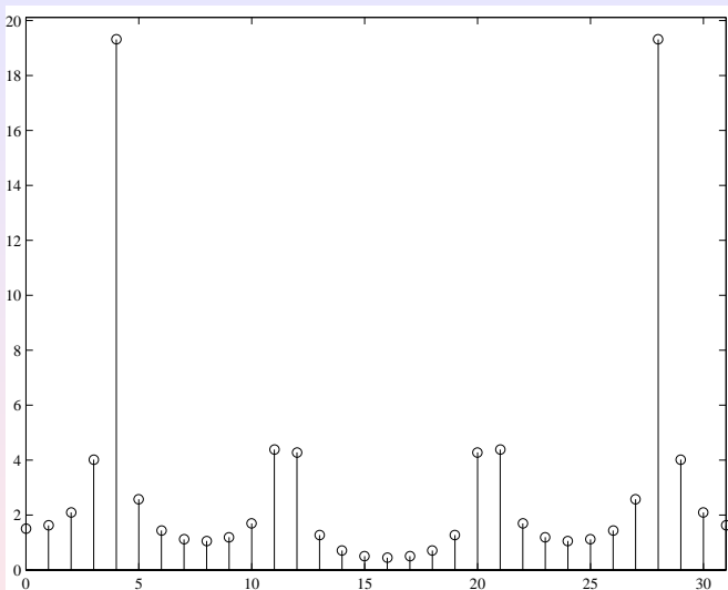
Slika: Spektar signala uz N = 32 , frekvencijska os u uzorcima DFT-a.
