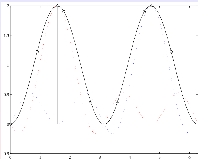
Slika: Realni dio spektra za P = L = 4 , N = 7
