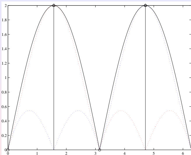
Slika: Amplitudni spektar (DFT i DTFT) za P = L = N = 4
