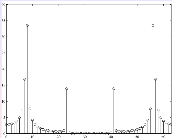
Slika: Spektar signala uz N = 64 , frekvencijska os u uzorcima DFT-a.
