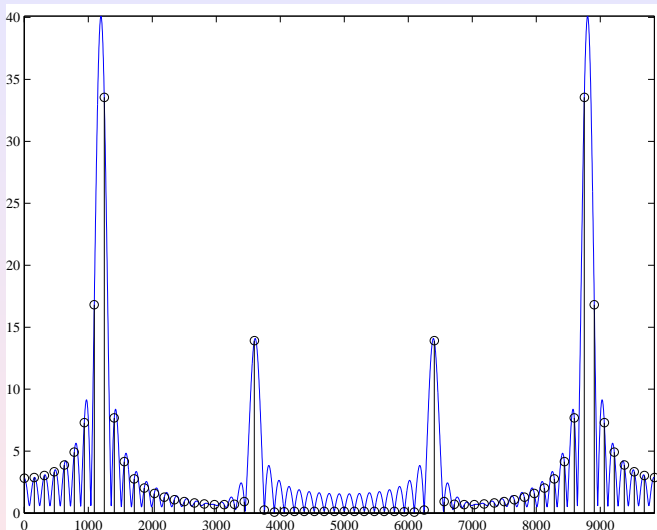
Slika: Spektar signala uz N = 64 , frekvencijska os u Hz.
