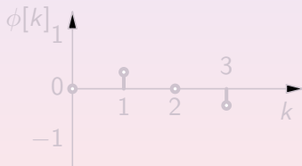
Slika: Amplitudni spektar
