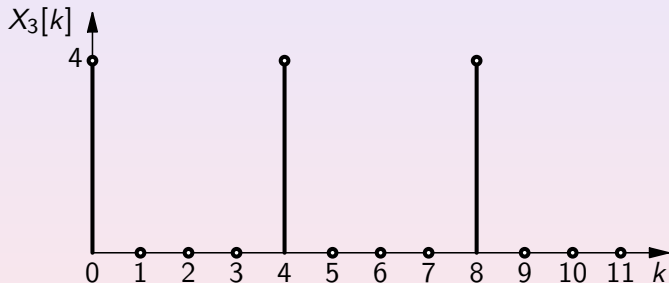
Slika: Amplitudni spektar X_3[k]
