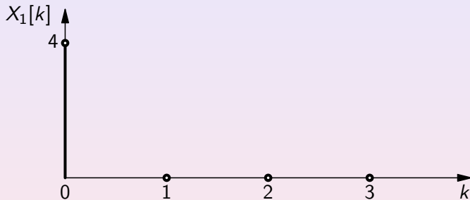
Slika: Amplitudni spektar X_1[k]
